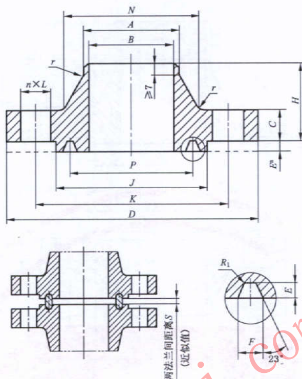
图 11 环连接面(RJ)对焊钢制管法兰
